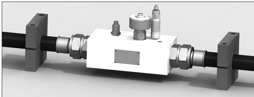
Présentation d'un débitmètre CT dans son montage type avec les options capteur de pression et capteur de température montées.
