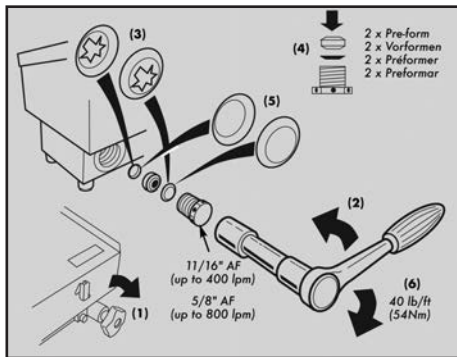
Esquema de sustitución de discos rotos. Nota: se muestra el comprobador DHM. El procedimiento para el modelo CTR es igual.
